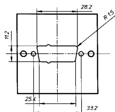
Målskisse
