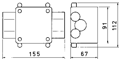
Målskisse
