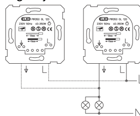
Koblingsskjema
