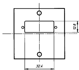
Målskisse
