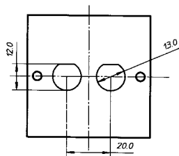
Målskisse
