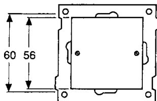
Målskisse
