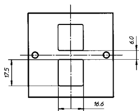
Målskisse
