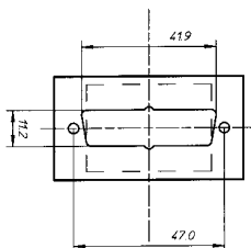
Målskisse
