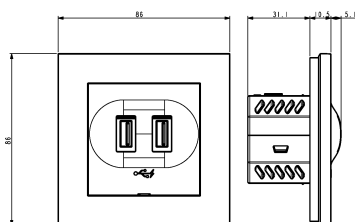
Målskisse
