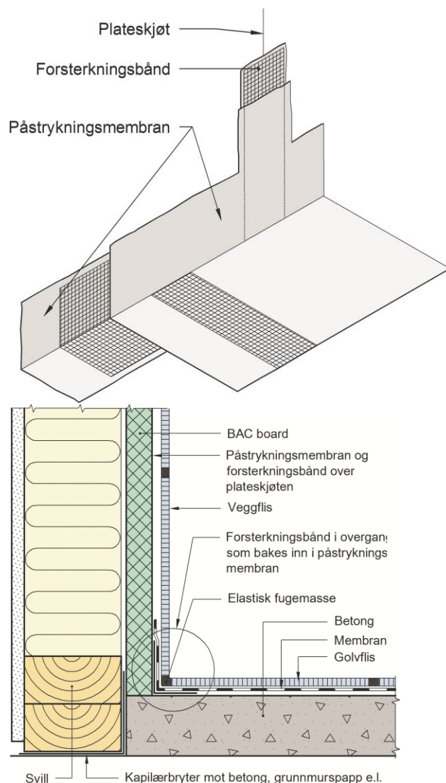
Fig. 3 Eksempel på overgang mellom flisdekket gulv og vegg med membran under flisene på gulv.
