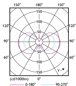
LEDcapsule G9
