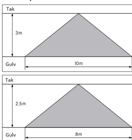
Takmontasje
