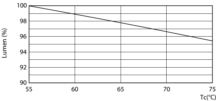
TLED_220-240V_G13-LumenVsTc
