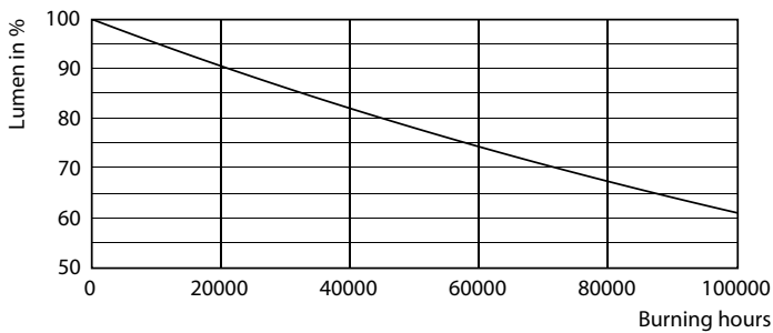
TLED_220-240V_G13
