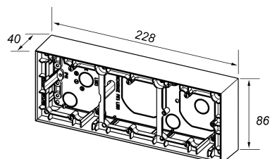
Målskisse
