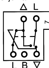
Koblingsskjema
