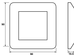
Målskisse
