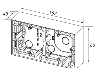
Målskisse
