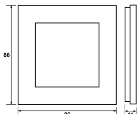
Målskisse
