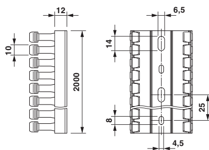
Målskisse
