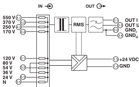
Blokkskjema
