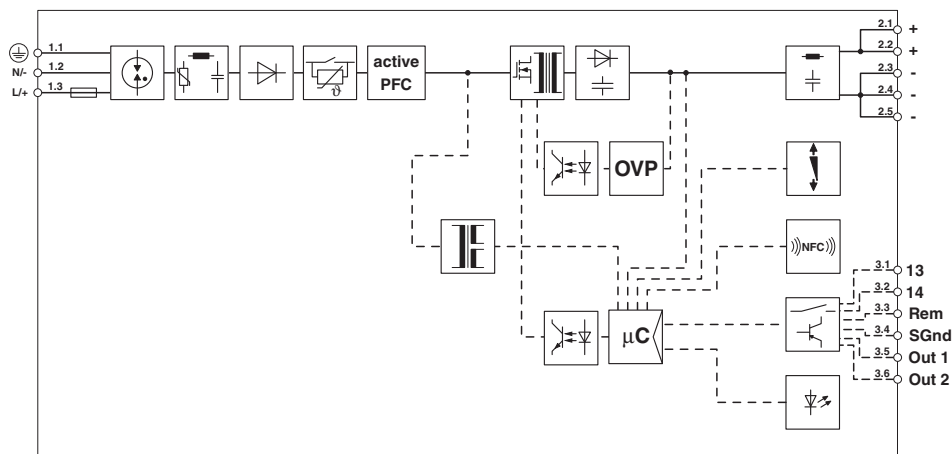
Blokkskjema
