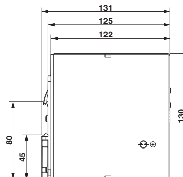
Målskisse
