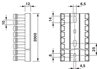
Målskisse
