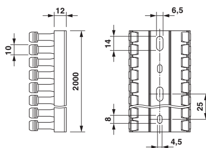
Målskisse
