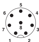
Skjemategning
