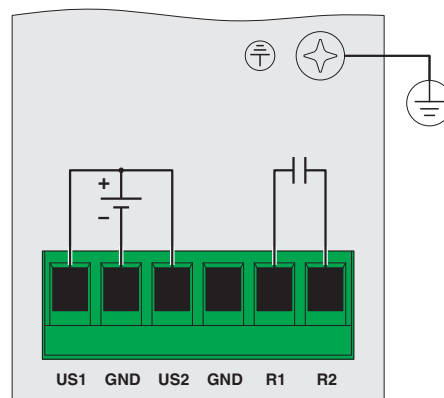
Tilkoblingstegning
