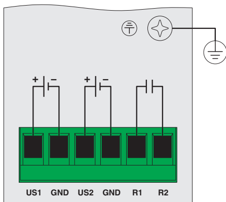
Tilkoblingstegning
