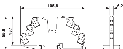
Målskisse
