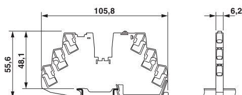
Målskisse
