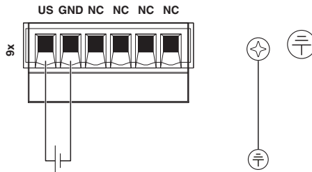
Tilkoblingstegning
