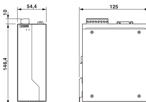
Målskisse
