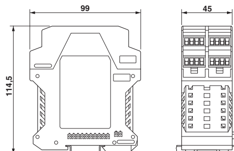
Målskisse
