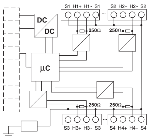
Blokkskjema
