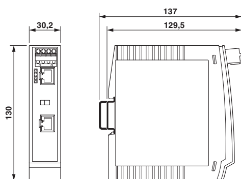
Målskisse
