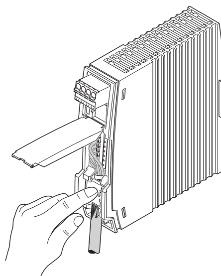
Lukk skjermkontaktfjær
