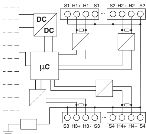
Blokkskjema
