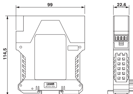
Målskisse
