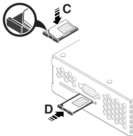
Legg inn SIM-kort
