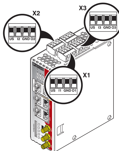
Tilkobling av ledningene
