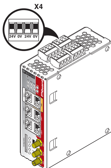
Tilkobling av forsyningsspenningen
