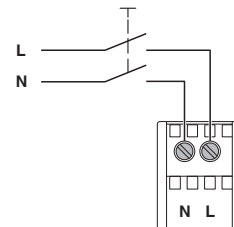
Tilkobling av forsyningsspenningen
