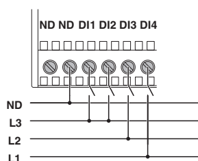
Tilkoblingstegning
