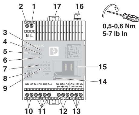
Frontvisning
