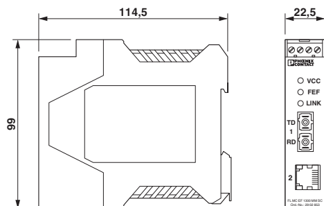
Målskisse
