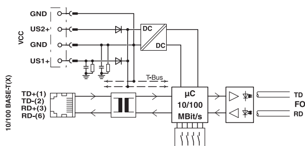
Blokkskjema
