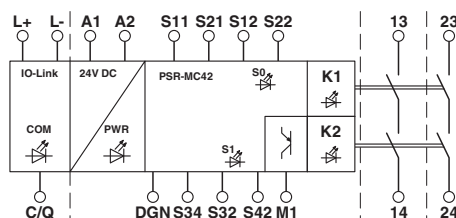
Blokkskjema
