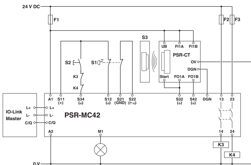
Koblingsskjema
