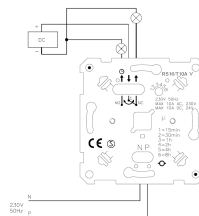
Koblingsskjema
