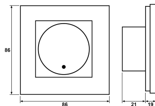
Målskisse
