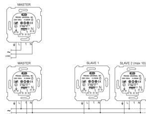
Koblingsskjema
