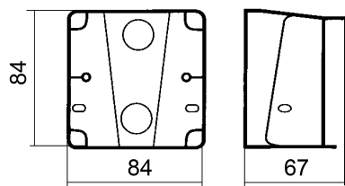
Målskisse
