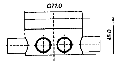
Målskisse
