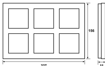
Målskisse
