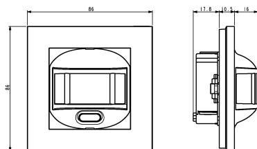
Målskisse
