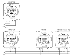
Koblingsskjema
