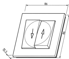
Målskisse
