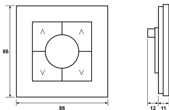
Målskisse
