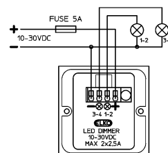
Koblingsskjema
