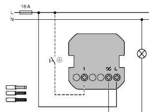
Koblingsskjema
