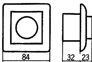
Målskisse
