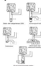
Koblingsskjema
