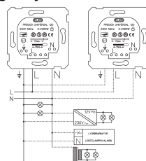
Koblingsskjema
