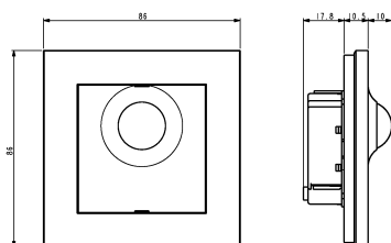
Målskisse
