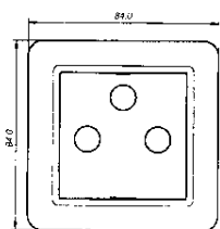
Målskisse
